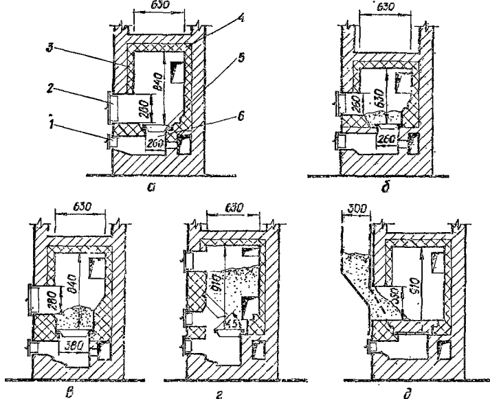
Рис. 12. Конструкции топливников:
