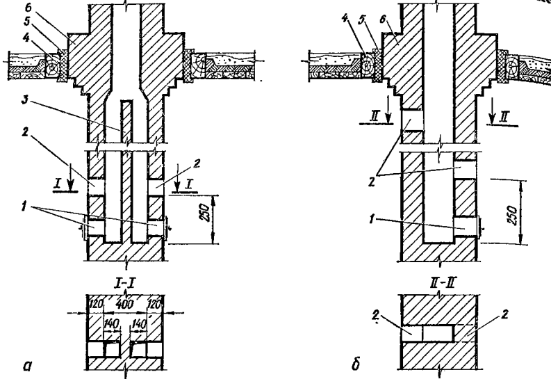
Рис. 45. Подключение двух печных устройств к одному дымовому каналу:
