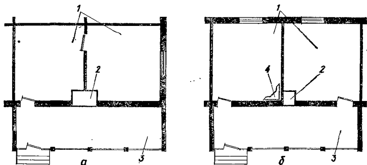
Рис. 17. Размещение печи ( a ), а также печи и камин ( б ) в зданиях дачного или садового типа:
