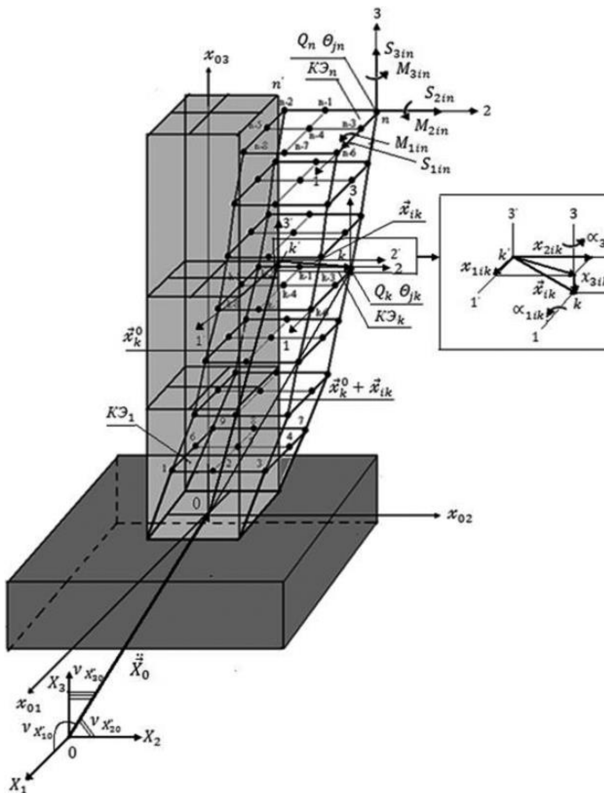
Рисунок 7.1 - i -я форма колебаний пространственной РДМ
