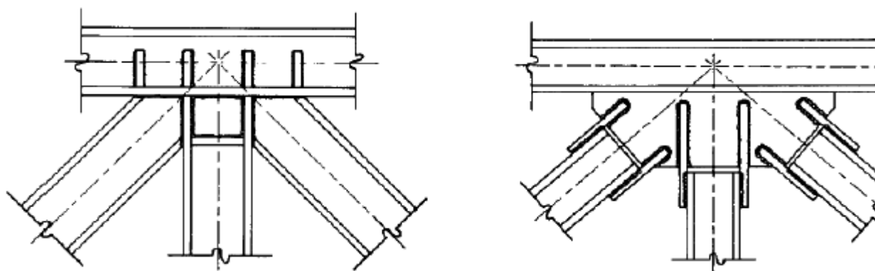
Рисунок Б.2 - Примеры выполнения узлов аутригерных ферм
