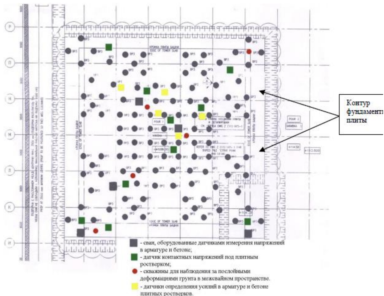
Рисунок В.1 - Пример схемы размещения датчиков при геотехническом мониторинге строящегося высотного здания
