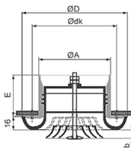
Рисунок 1 - Конструктивная схема диффузора веерного
