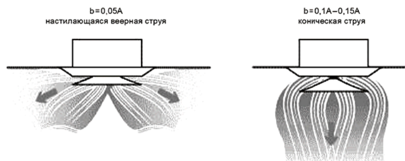
Рисунок 2 - Схемы струй, формируемых диффузором
