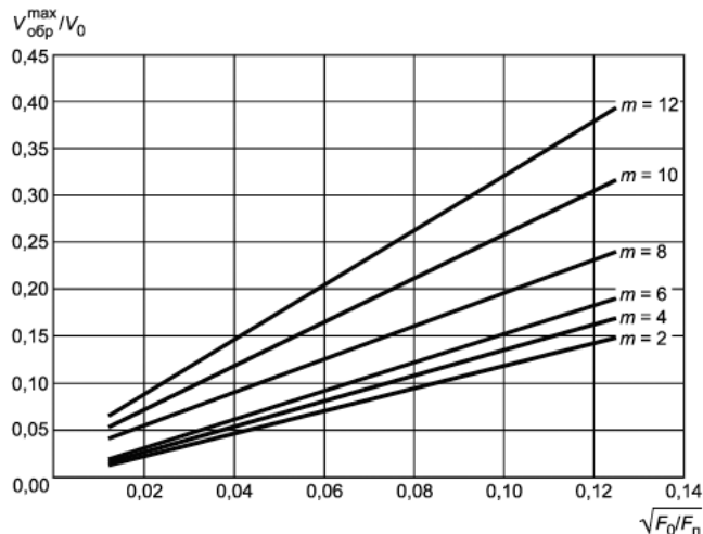
Рисунок Ж.2 - Зависимость максимальной скорости в обратном потоке от параметра \sqrt{F_0/F_n} стеснения и кинематического коэффициента m ВР
