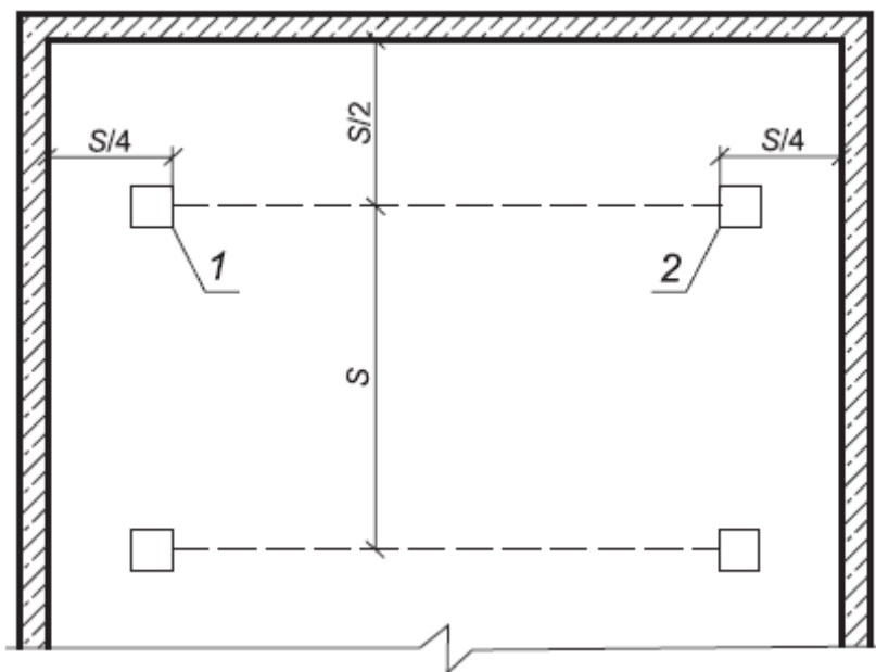
Рисунок Г.2 - Графический материал к требованиям 6.6.18
