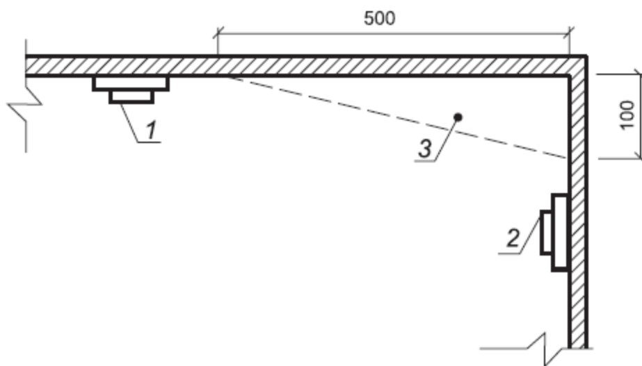
Рисунок Г.1 - Графический материал к требованиям 6.6.9 и 6.6.36
