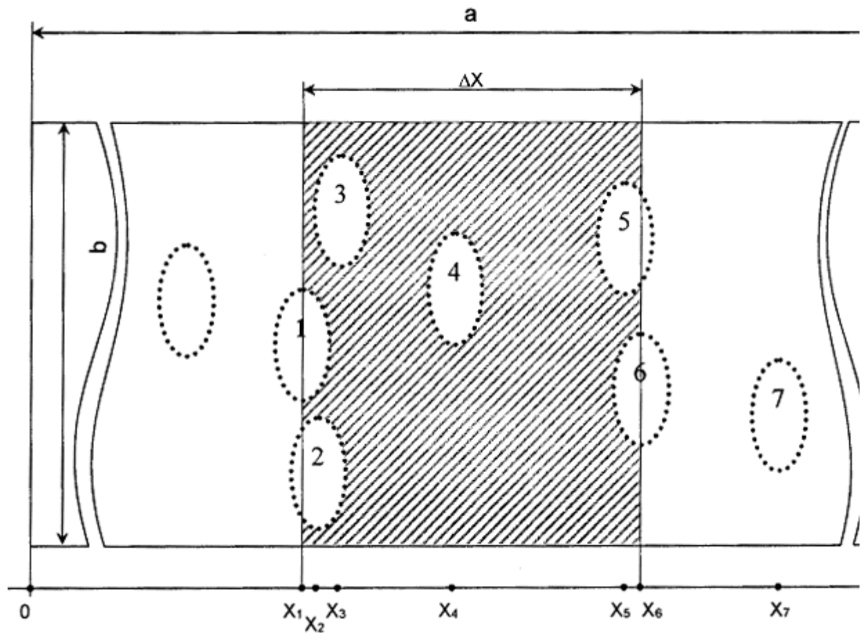
Рисунок П7.1. Координатная схема размещения людей на путях эвакуации
