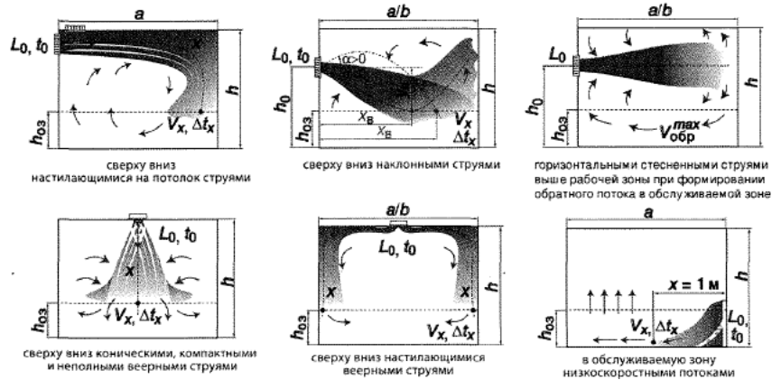
Рисунок Л.1 - Основные схемы подачи приточного воздуха
