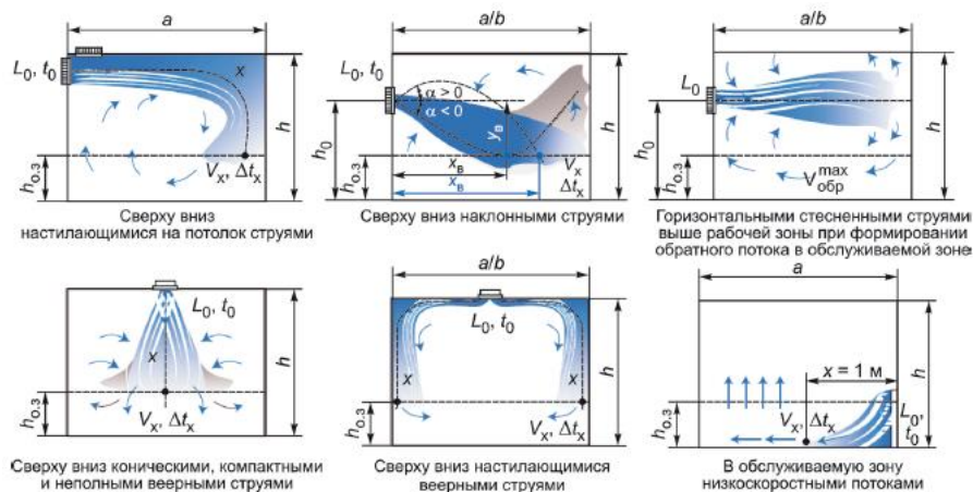
Рисунок Ж.1 - Основные схемы подачи приточного воздуха
