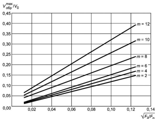
Рисунок Ж.2 - Зависимость максимальной скорости в обратном потоке от параметра стеснения и кинематического коэффициента m ВР
