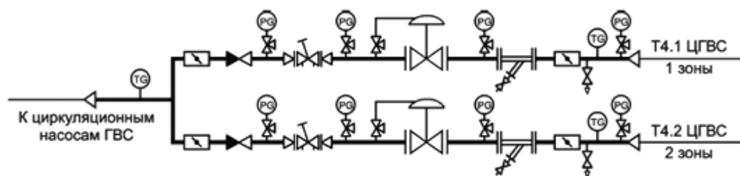
Рисунок 5.8 - Узел регулирования давления и расхода в циркуляционных трубопроводах двухзонной схемы горячего водоснабжения
