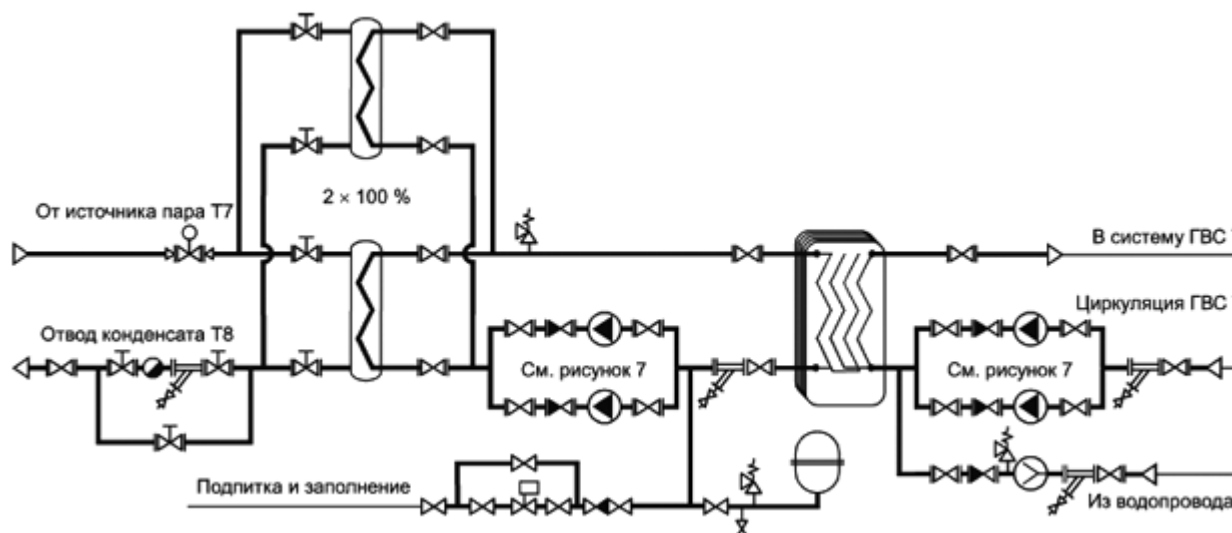
Рисунок 5.10 - Блок горячего водоснабжения с промежуточным контуром при T_{\text{п}} < 150^{\circ}\text{C}
