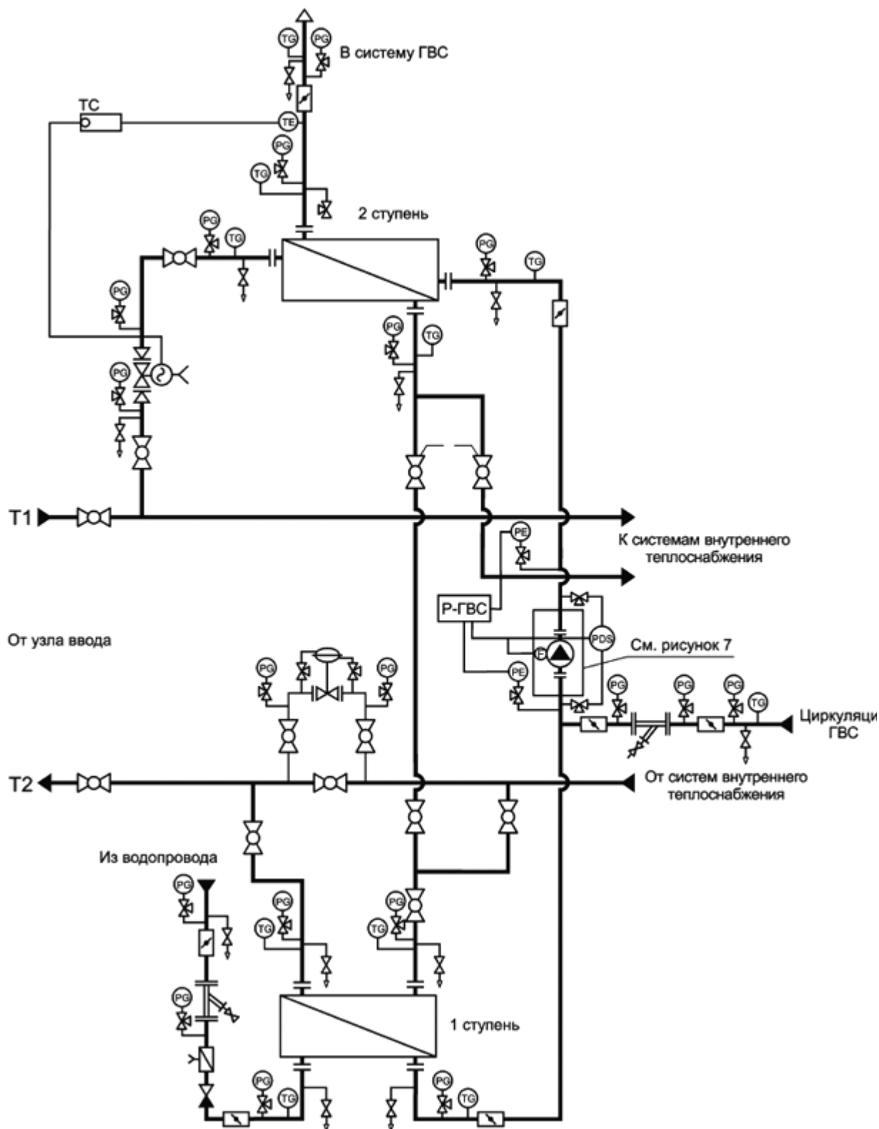
Рисунок 5.4 - Двухступенчатая циркуляционно-повысительная схема горячего водоснабжения
