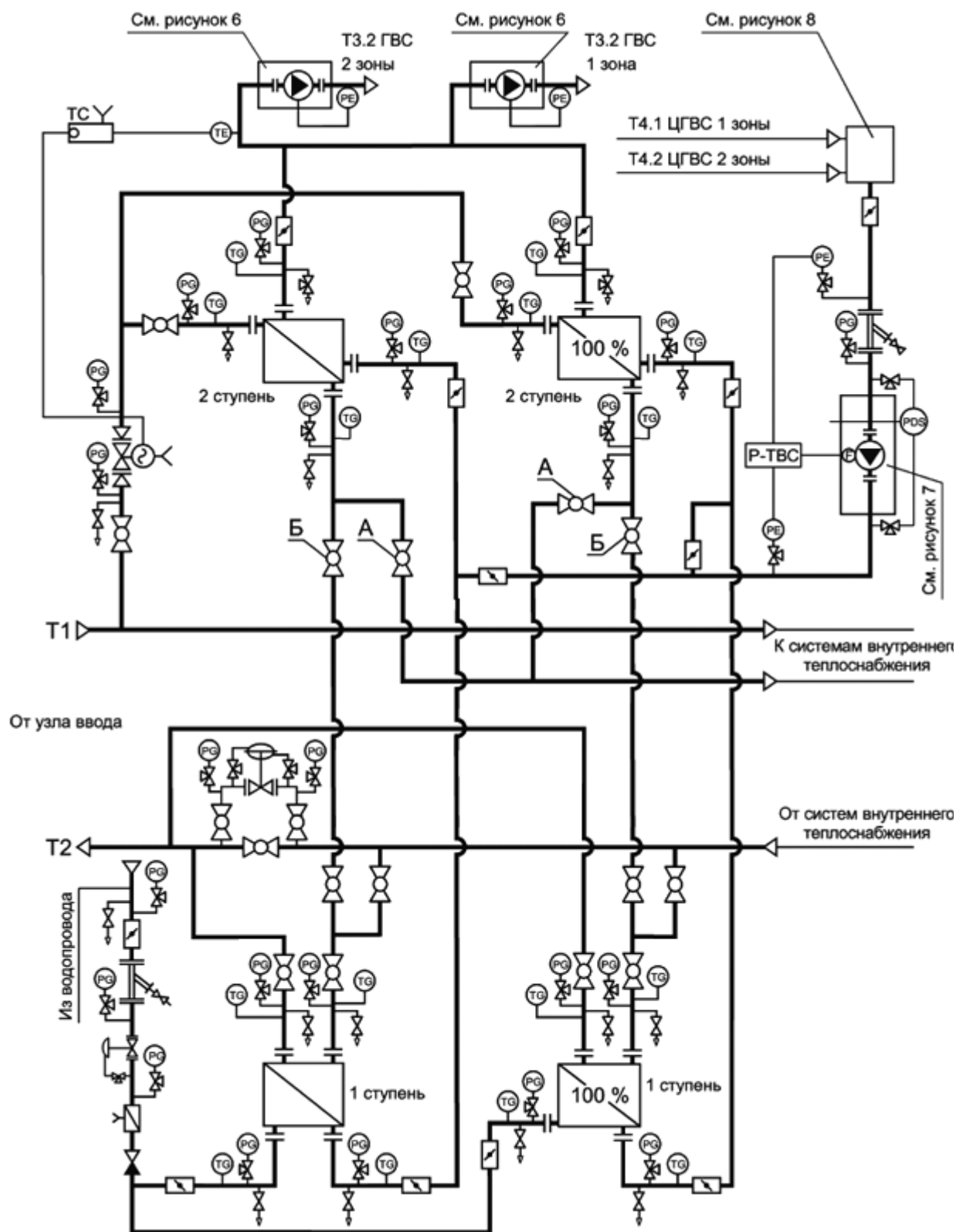
Рисунок 5.5 - Двухступенчатая схема горячего водоснабжения здания с двумя зонами по высоте
