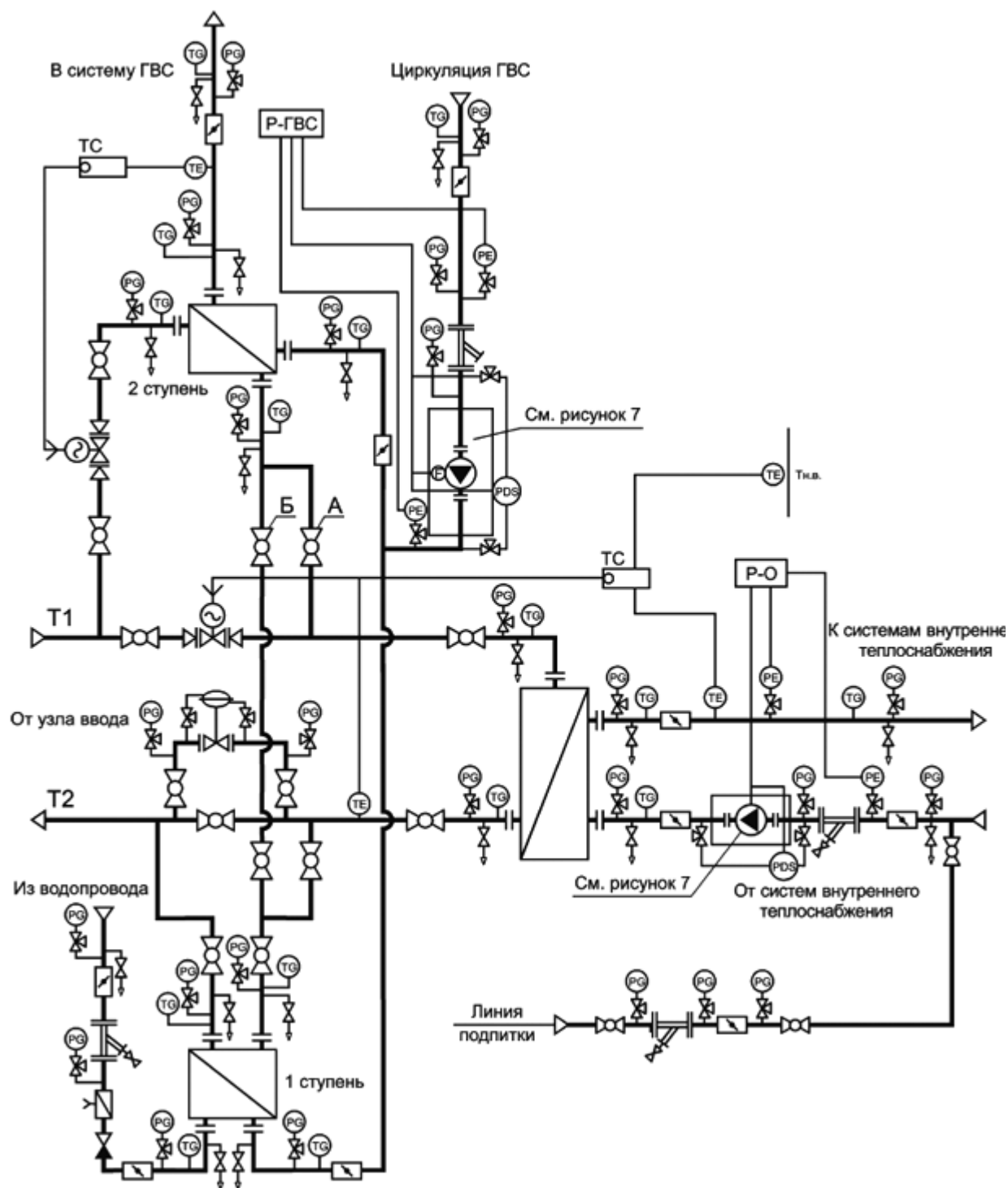
Рисунок 5.3 - Двухступенчатая схема горячего водоснабжения с независимым присоединением систем отопления (вентиляции)
