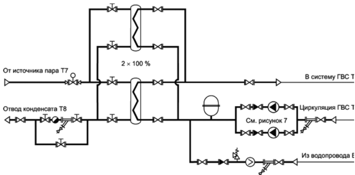
Рисунок 5.9 - Блок горячего водоснабжения с промежуточным контуром при T_{п} \geq 150^{\circ}\text{C}
